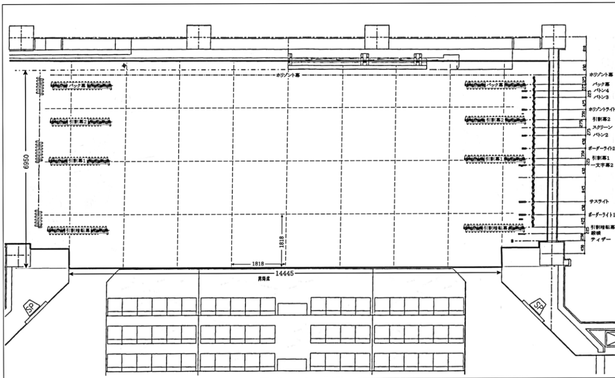
中央公民館ホール舞台平面図 (反響板なし)
