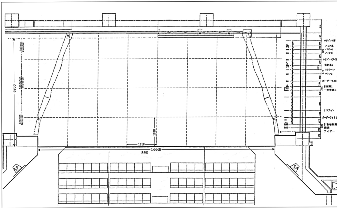
中央公民館ホール舞台平面図 (反響板あり)
