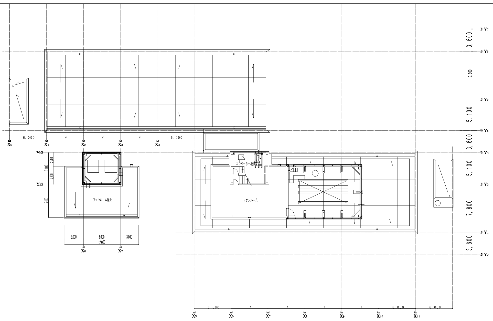
北棟R階平面図
