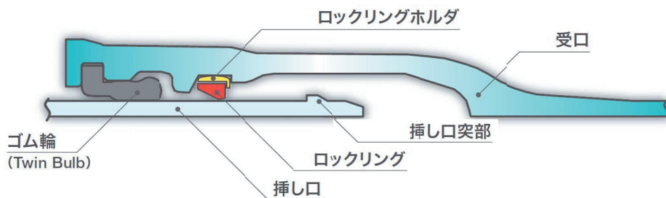
GX形ダクタイトイル鉄管の継手断面図
