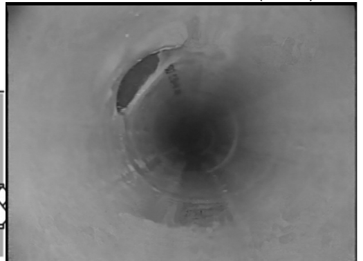
更生工事施工後の管渠(参考)
