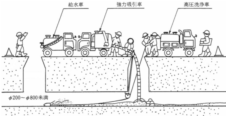
下水管更生工事 作業図
